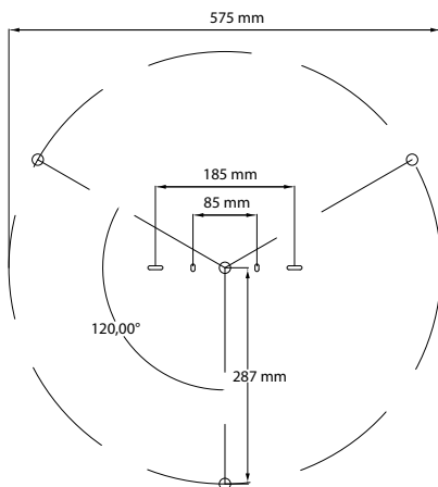
Dima per foratura dei cavi di sospensione e del rosone Drilling template for suspension cables and ceiling rose
